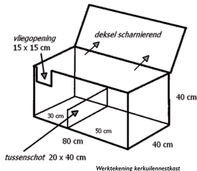
Werktekening kerkuilennestkast
